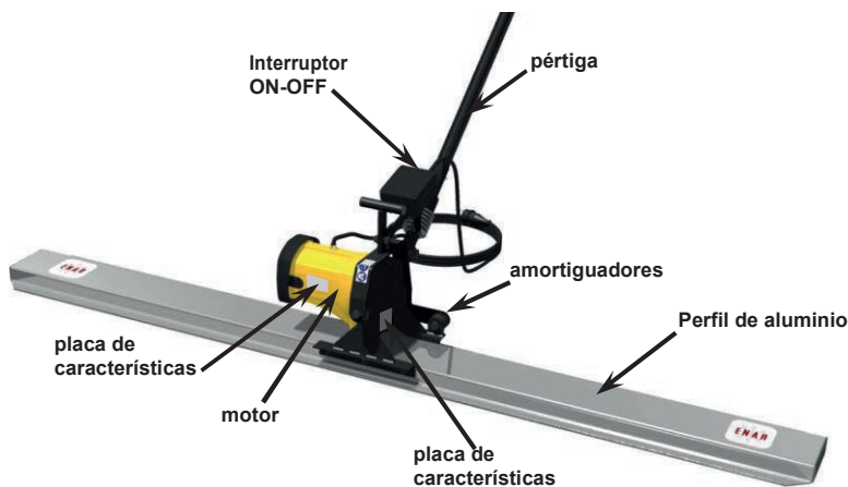
REGLAS VIBRO-EXTENDEDORAS OSCILANTES CON MOTOR ELÉCTRICO O GASOLINA "QZ"
