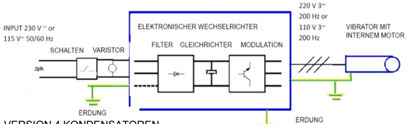
6.1 VERSION 4 KONDENSATOREN
